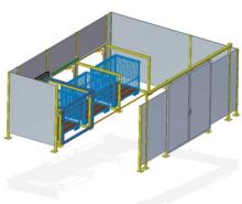
BIN-PICKING Roboterzelle mit 3 Kammern
